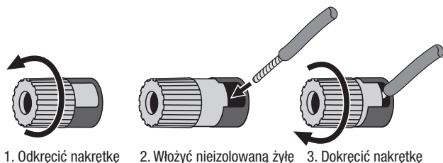
1. Odkręć nakrętkę 2. Włożyć nieizolowaną żyłę 3. Dokręć nakrętkę
